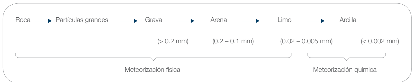
Figura 2. Proceso de degradación de la roca.
