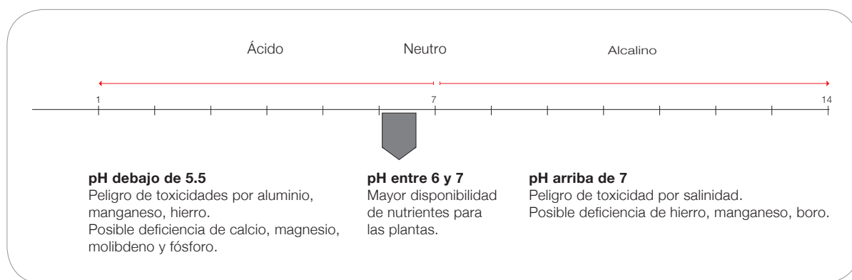
Figura 11. pH del suelo y la disponibilidad de nutrientes para las plantas.
