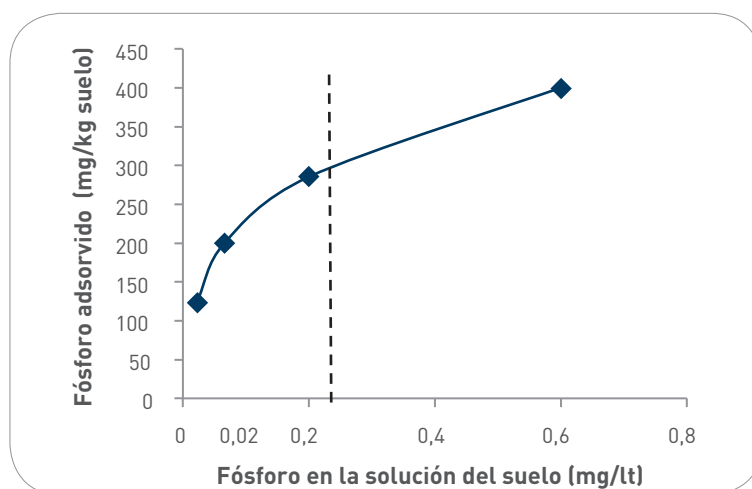
Figura 18. Relación entre el fósforo en solución y el adsorbido en un suelo arcilloso y altamente meteorizado de Carolina del Norte, Estados Unidos.
