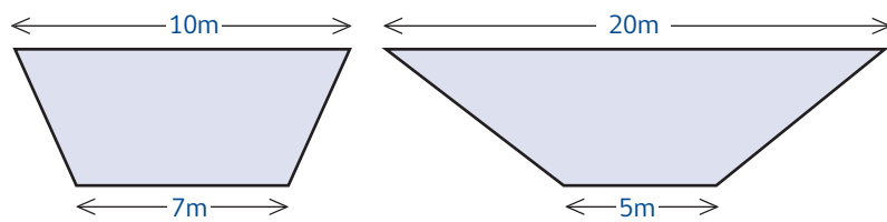
Cubicación de la capacidad de almacenamiento de una aguada superficial. (fotos: INIA)
