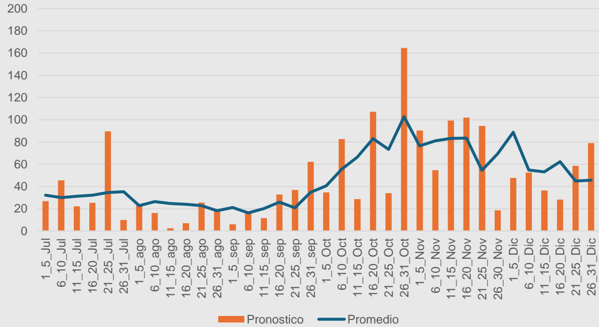
Pronostico de lluvias, cada 5 dias, Roatan, 2024
