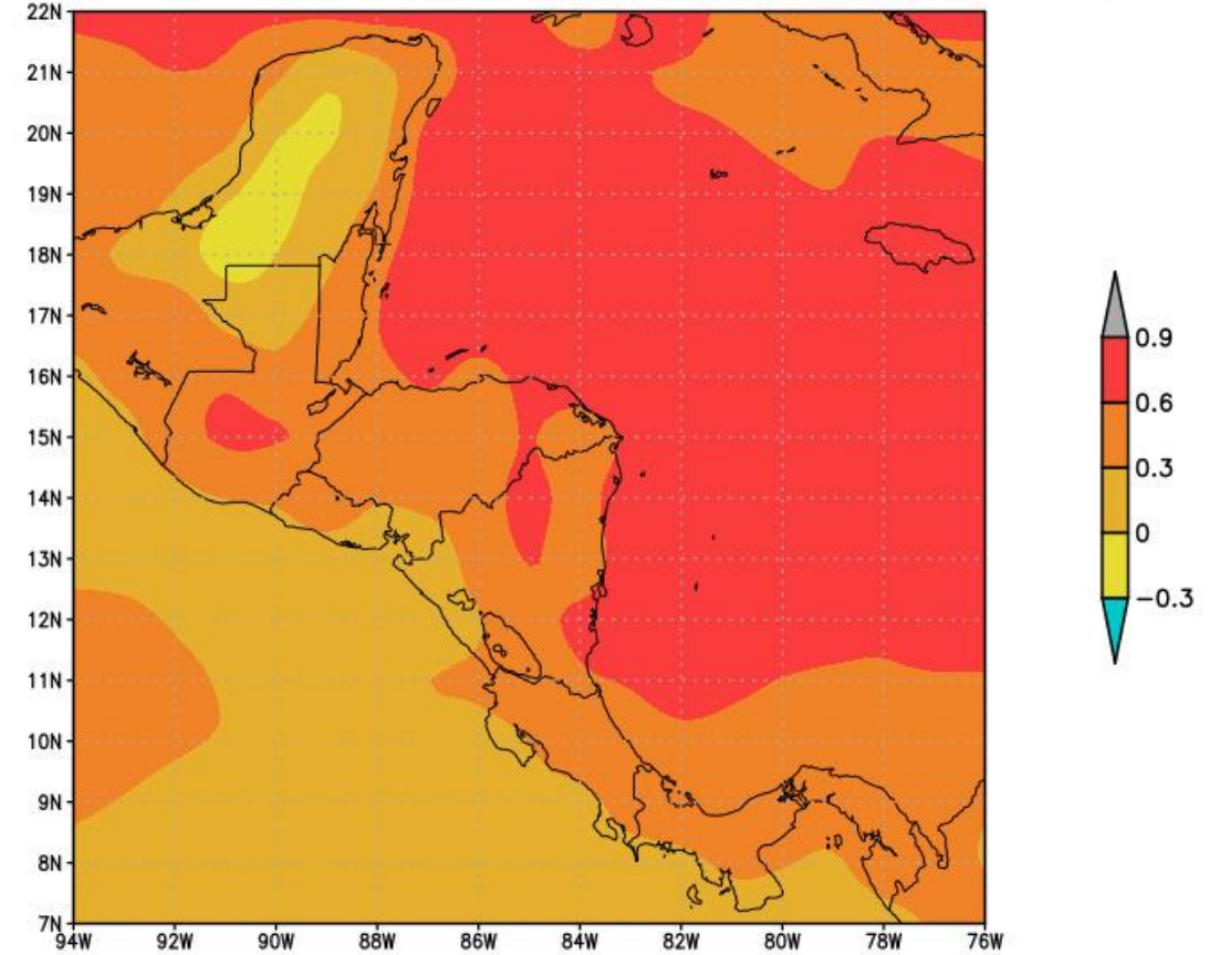
"Pronostico de anomalia de Temp. A-S-O 2024, NMME (gC)"
