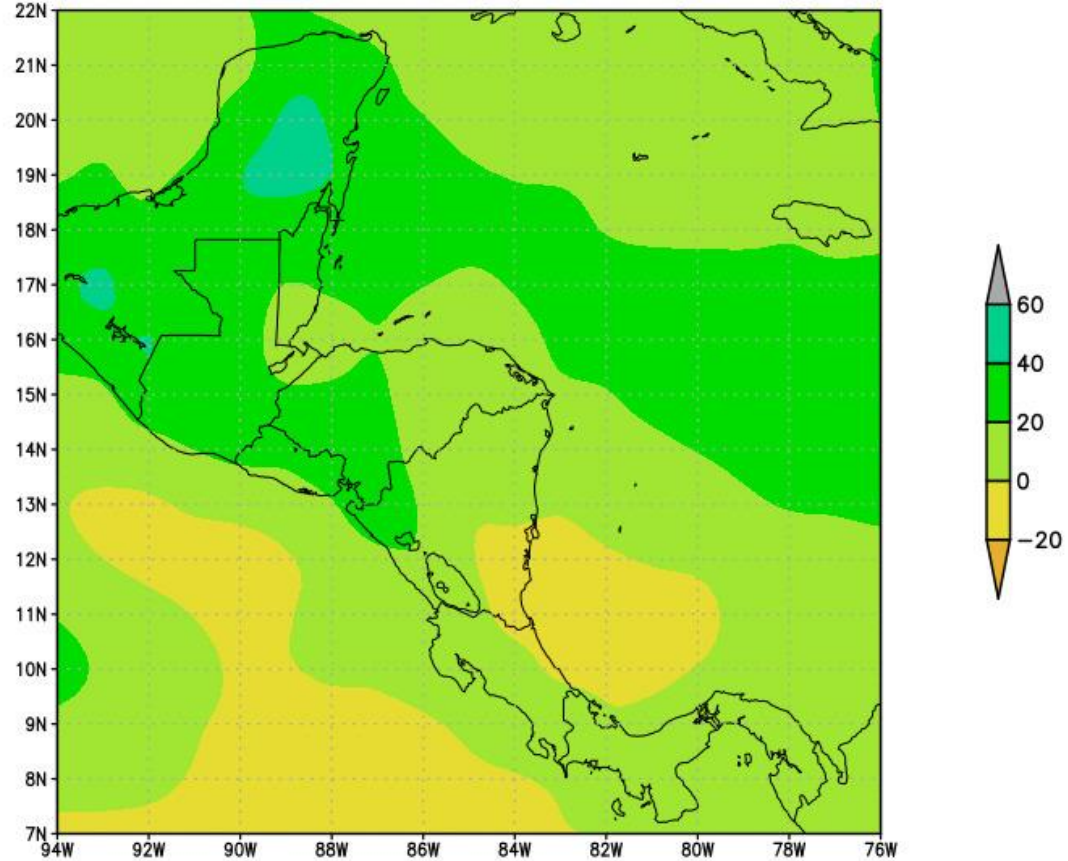
"pronostico de anomalia de lluvia en agosto 2024, NMME (%)"
