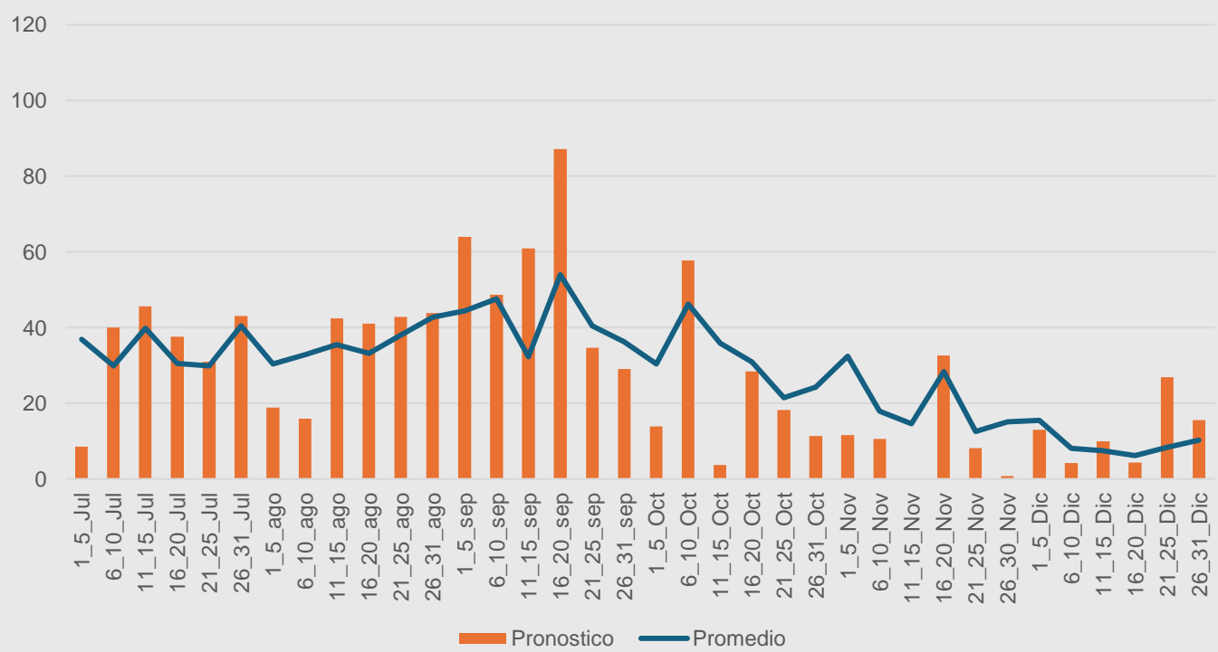
Pronostico de lluvia, cada 5 dias, Santa Barbara, 2024
