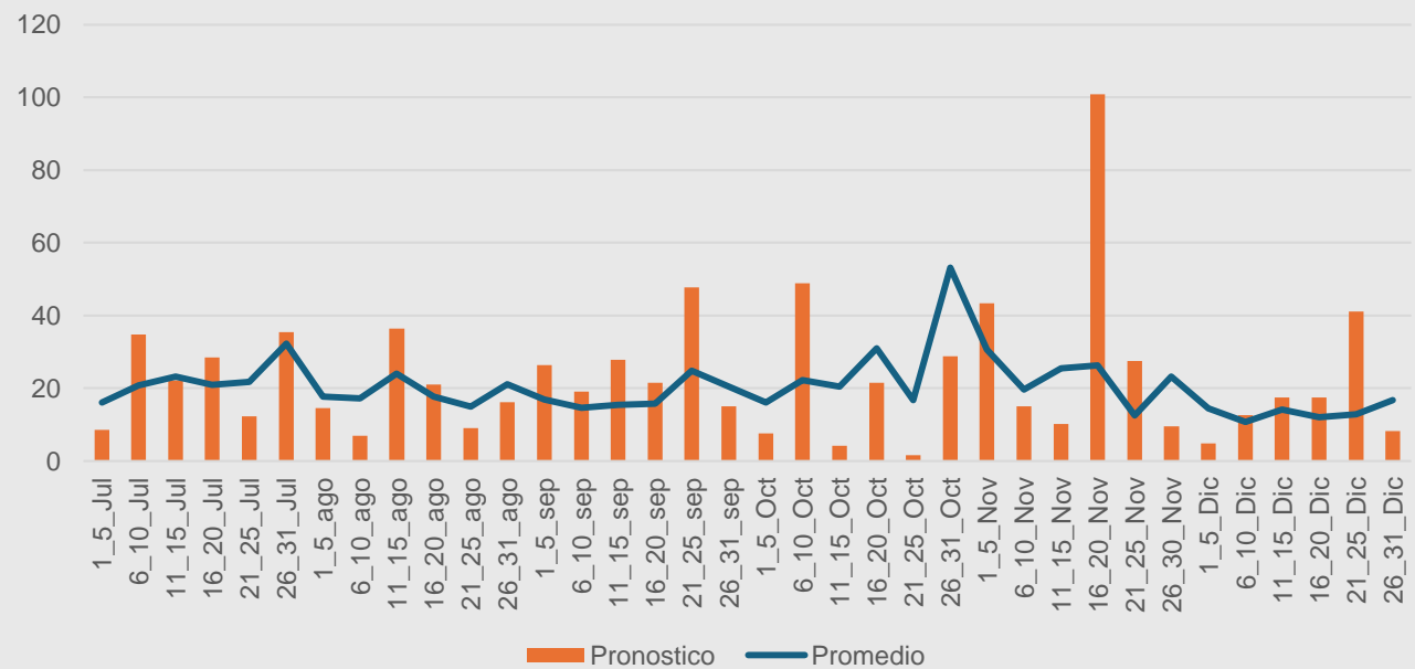
Pronostico de lluvia, cada 5 dias, Olanchito, 2024
