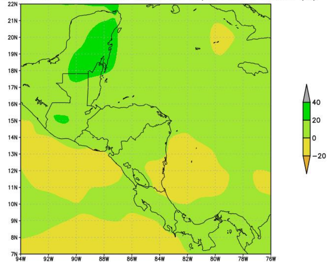
"pronostico de anomalia de lluvia en sept. 2024, NMME (%)"
