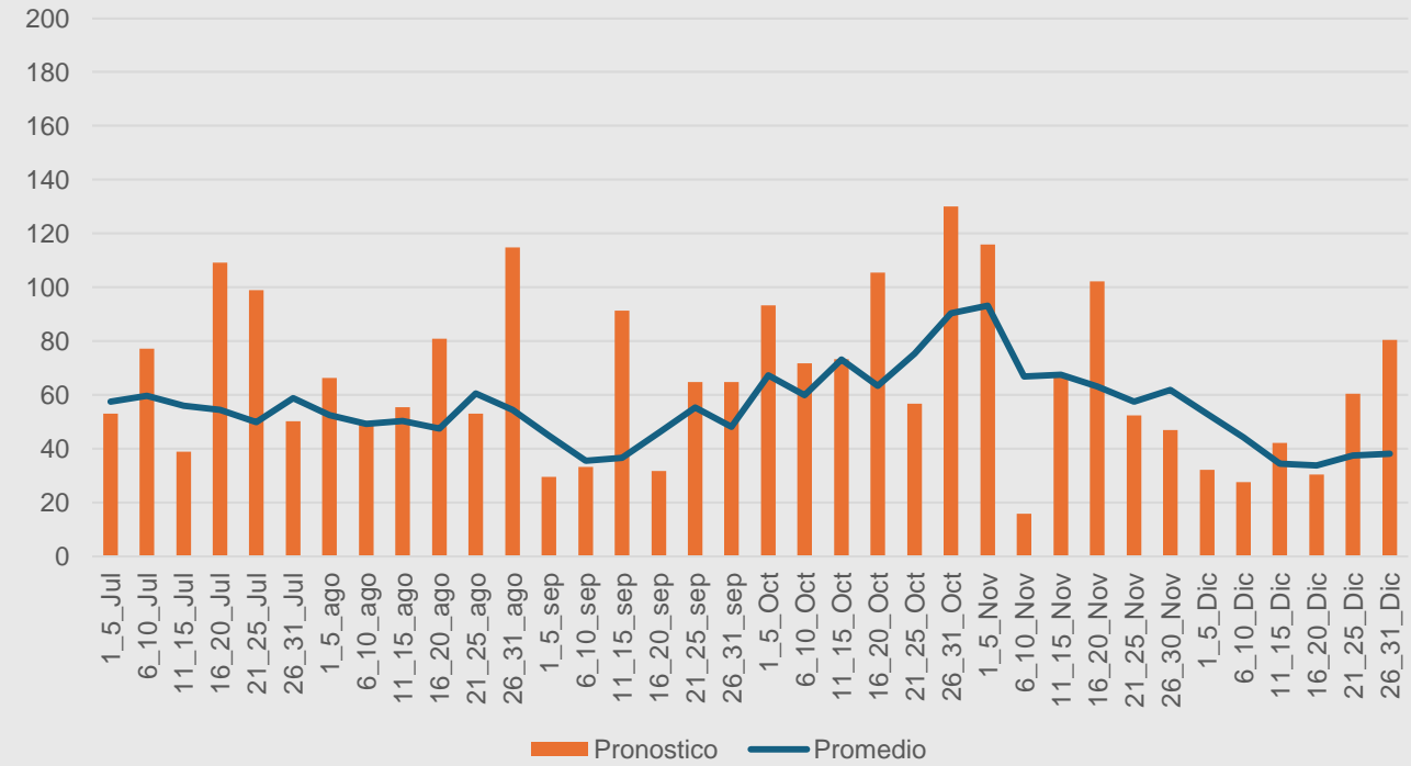
Pronostico de lluvia, cada 5 dias, Pto. Lempira, 2024
