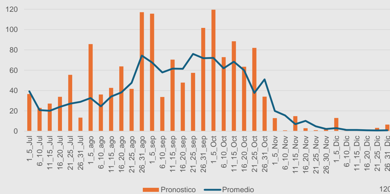
Pronostico de lluvias, cada 5 dias, Choluteca, 2024
