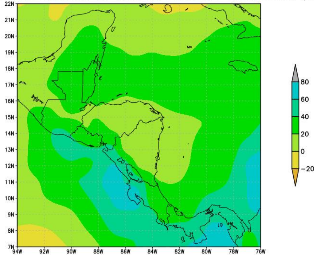
"pronostico de anomalia de lluvia en diciembre 2024, NMME (%)"
