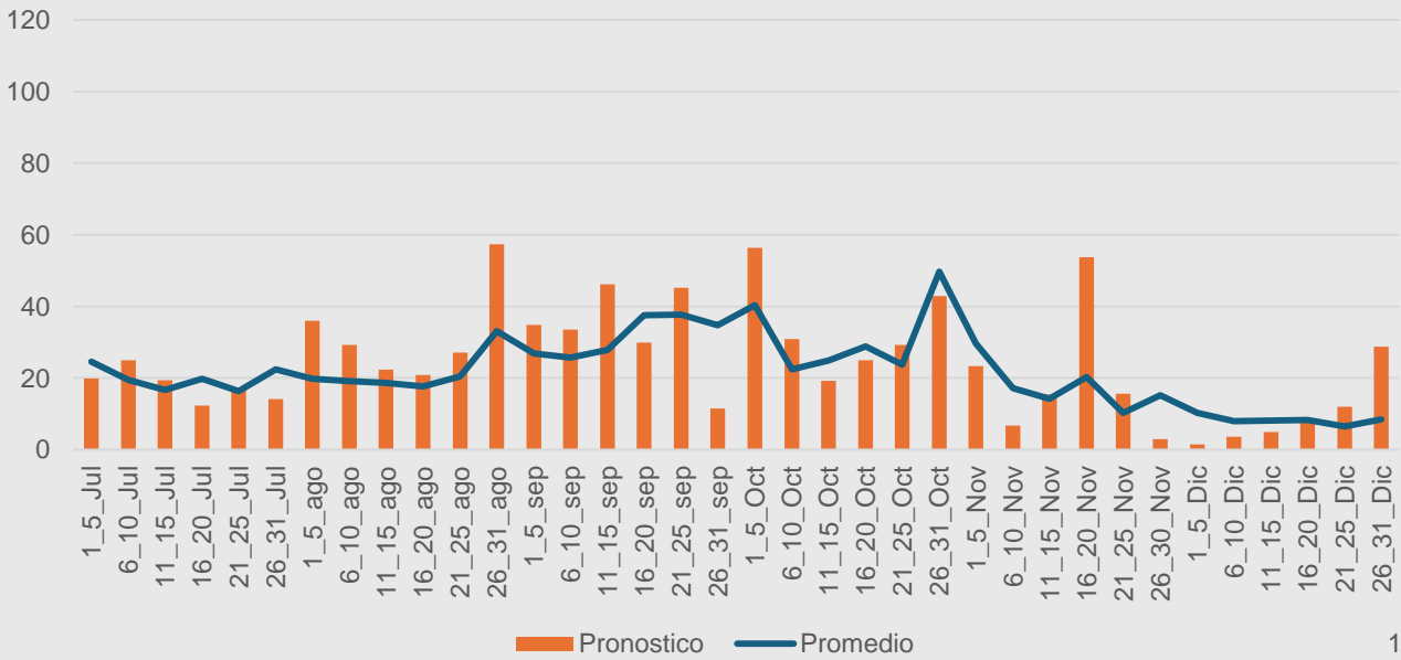
Pronostico de llluvias cada 5 dias de Yoro, 2024
