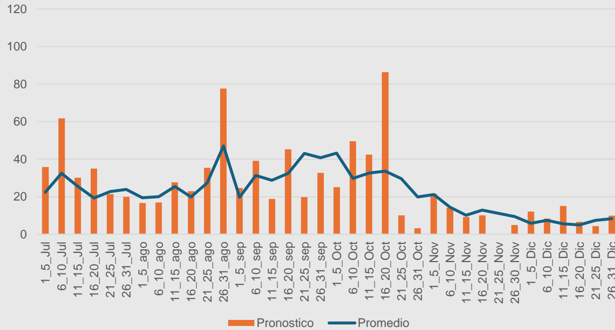
Pronostico de Lluvia, cada 5 idas, Lepaguare, 2024
