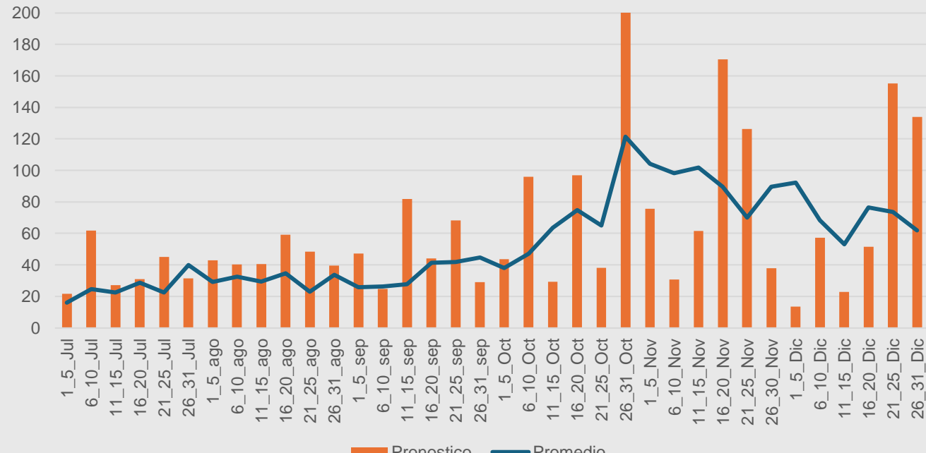
Pronostico de lluvias, cada 5 dias, La Ceiba, 2024
